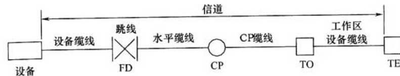
图 3.3.2 配线子系统缆线划分
