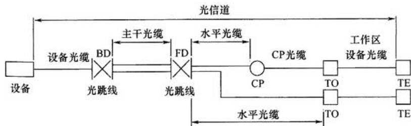
图 3.2.4-1 光纤信道构成 1
